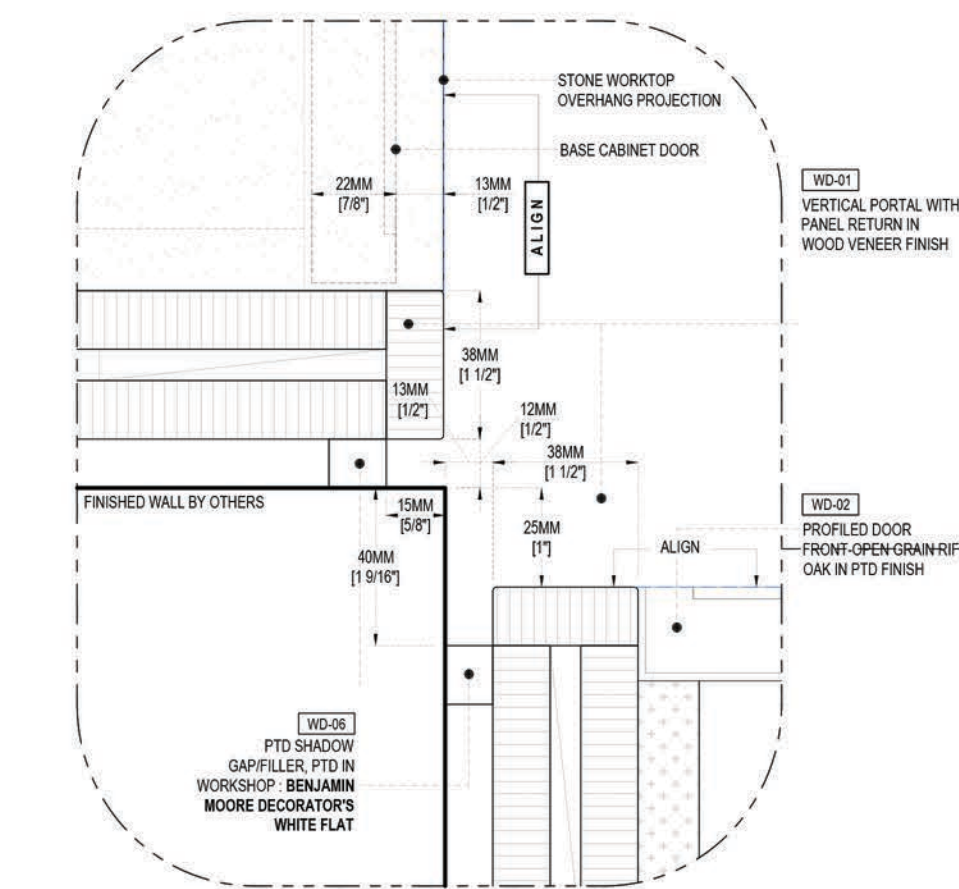
2 SCALE: 6" = 1'-0"
