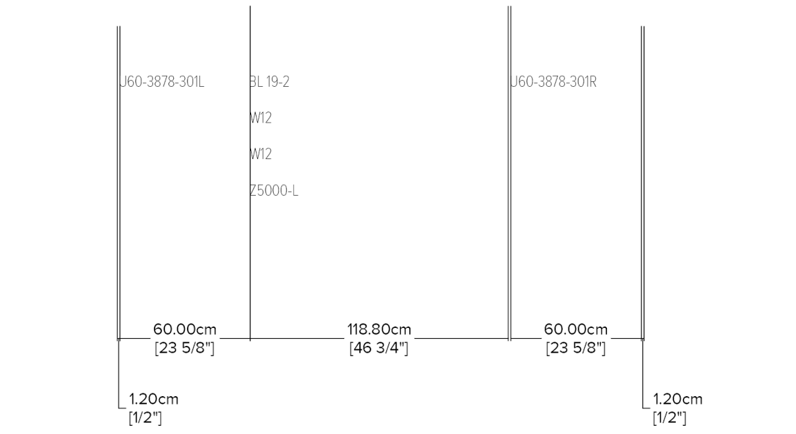
E ELEVATION
