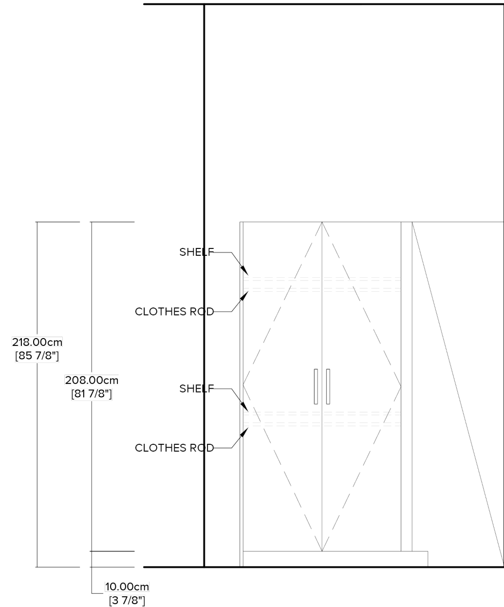
A ELEVATION
